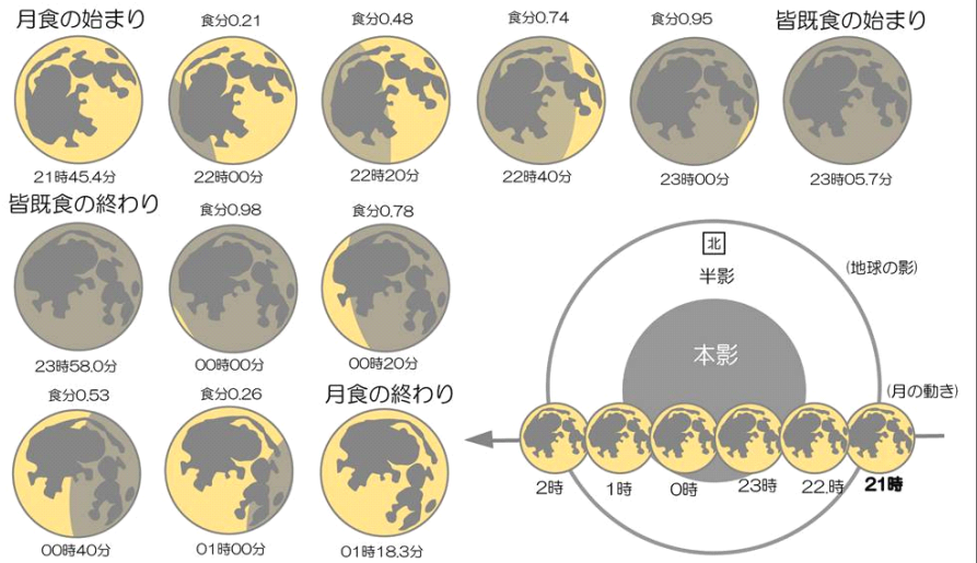
12月10日~11日の皆既月食のようす
