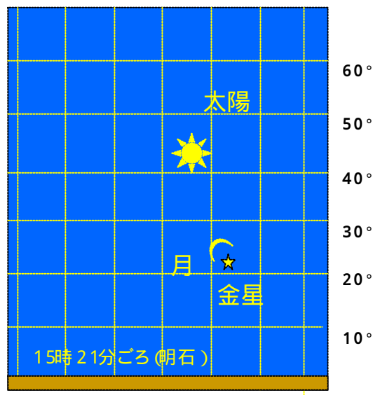
潜出（金星が月から出てくる）
