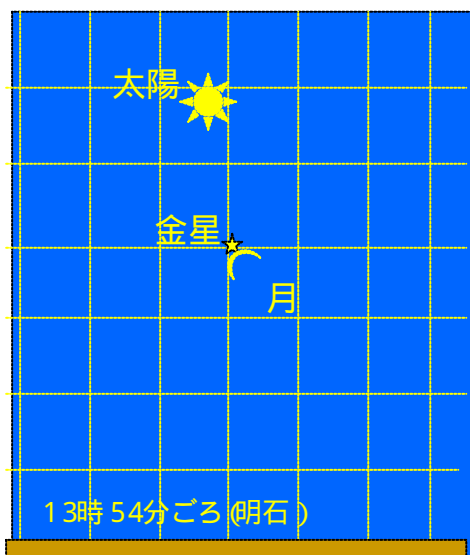
潜入（金星が月に隠れる）
