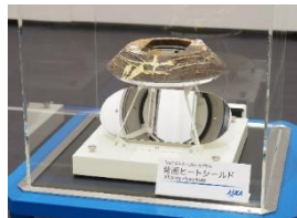
③背面ヒートシールド(実物)
